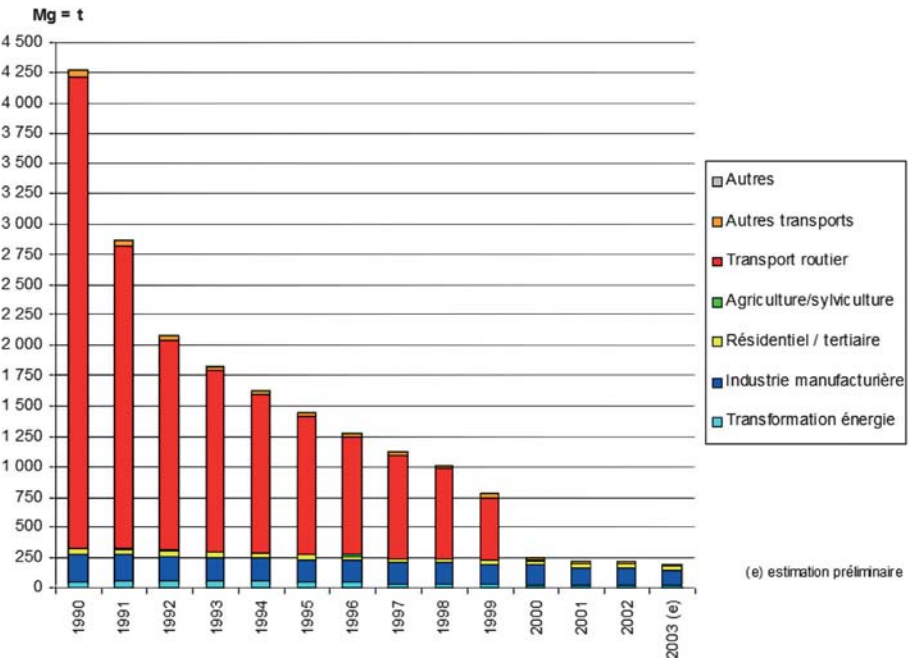
Figure 2.1 : Émissions de plomb dans l'air en France métropolitaine 1990-2003 (d'après CITEPA)
