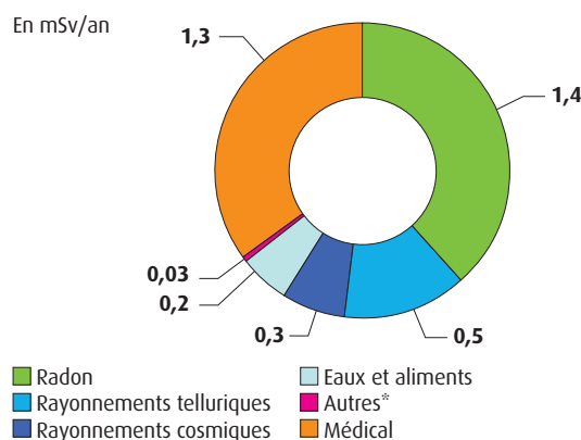
Figure 48 : exposition moyenne de la population aux rayonnements ionisants en France
