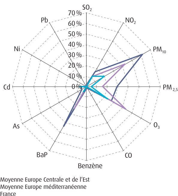
Figure 91 : taux de dépassement des seuils réglementaires par polluant en France, en Europe méditerranéenne et en Europe Centrale et de l'Est
