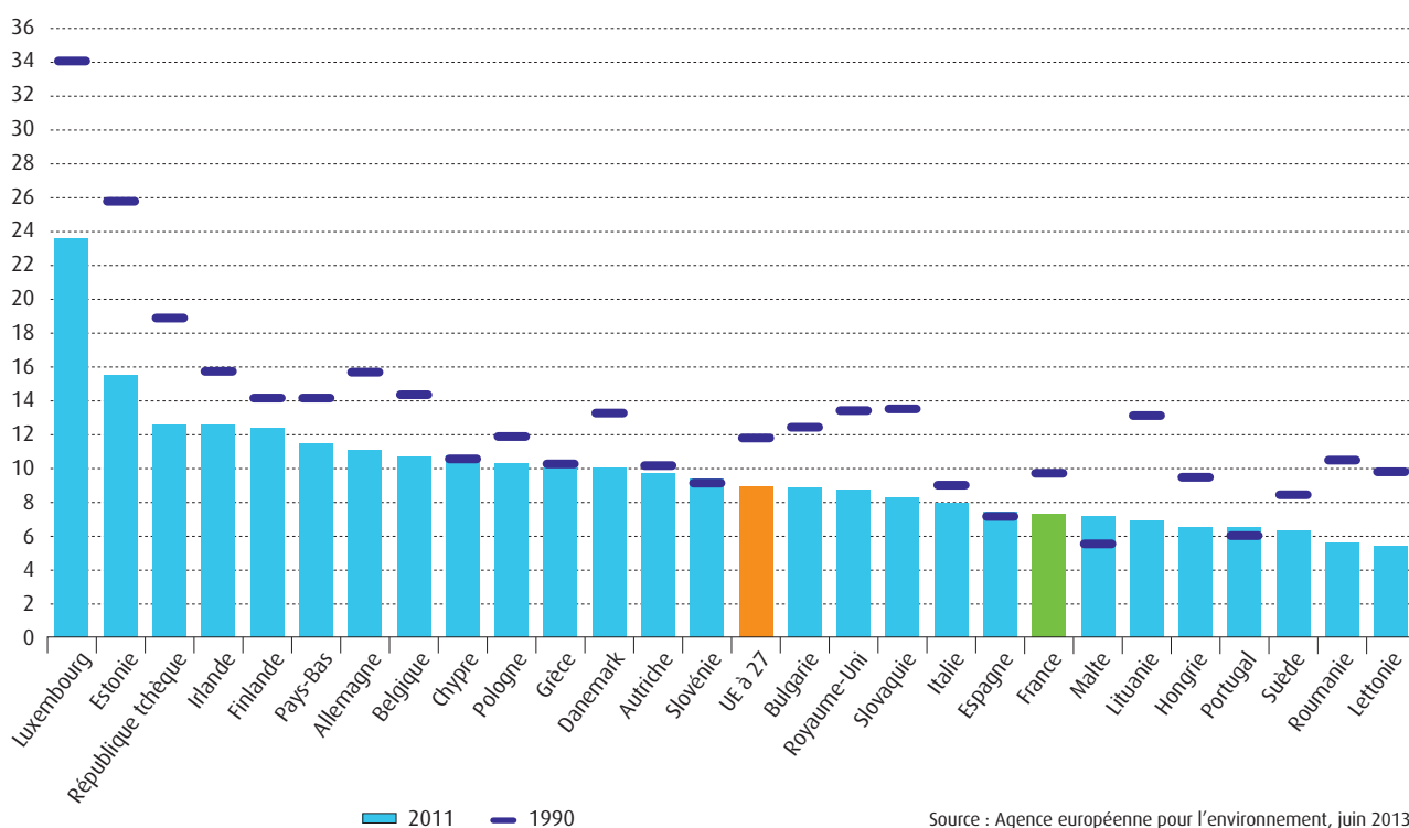
Figure 65 : évolution des émissions de GES par habitant dans l'Union européenne
