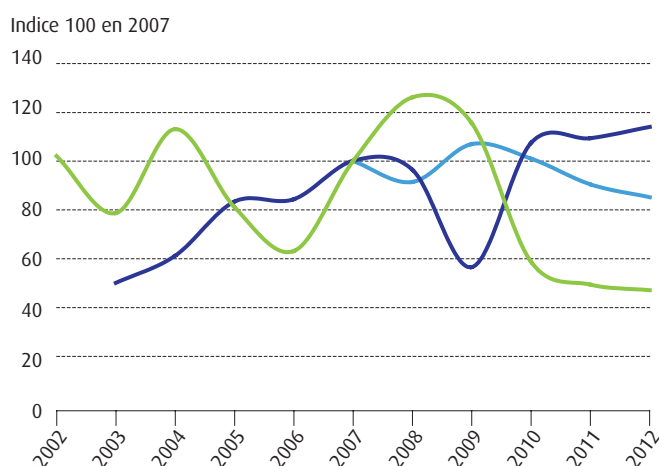
Figure 43 : évolution des blooms algaux dans les eaux métropolitaines
