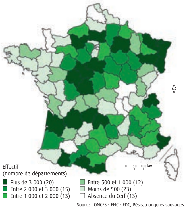
Figure 16 : répartition du Cerf élaphe en 2010
