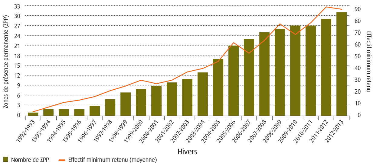
Figure 13 : évolution de la présence du Loup en France
