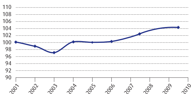
Figure 9 : évolution de l'indice poisson rivière
