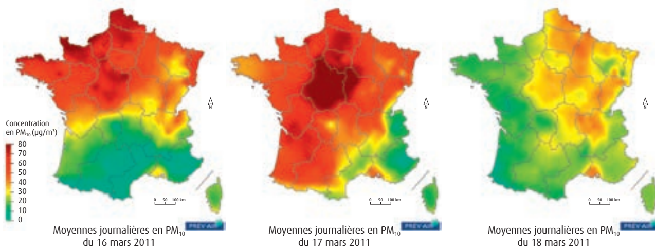
Figure 82 : épisode de pollution en particules \text{PM}_{10} en mars 2011
