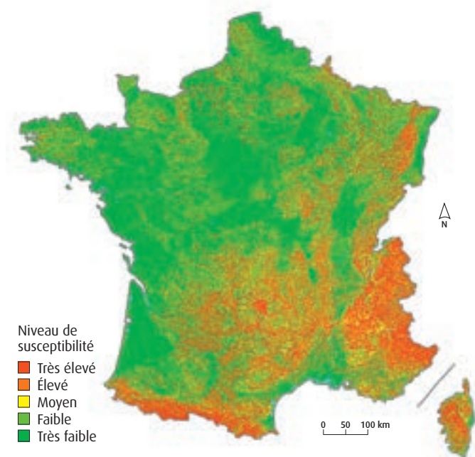
Figure 46 : susceptibilité des versants aux glissements de terrain
