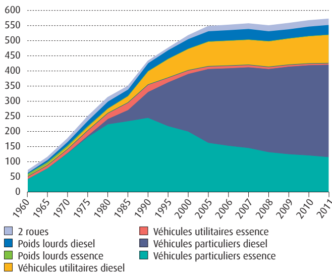
Figure 75 : évolution de la circulation par type de motorisation
