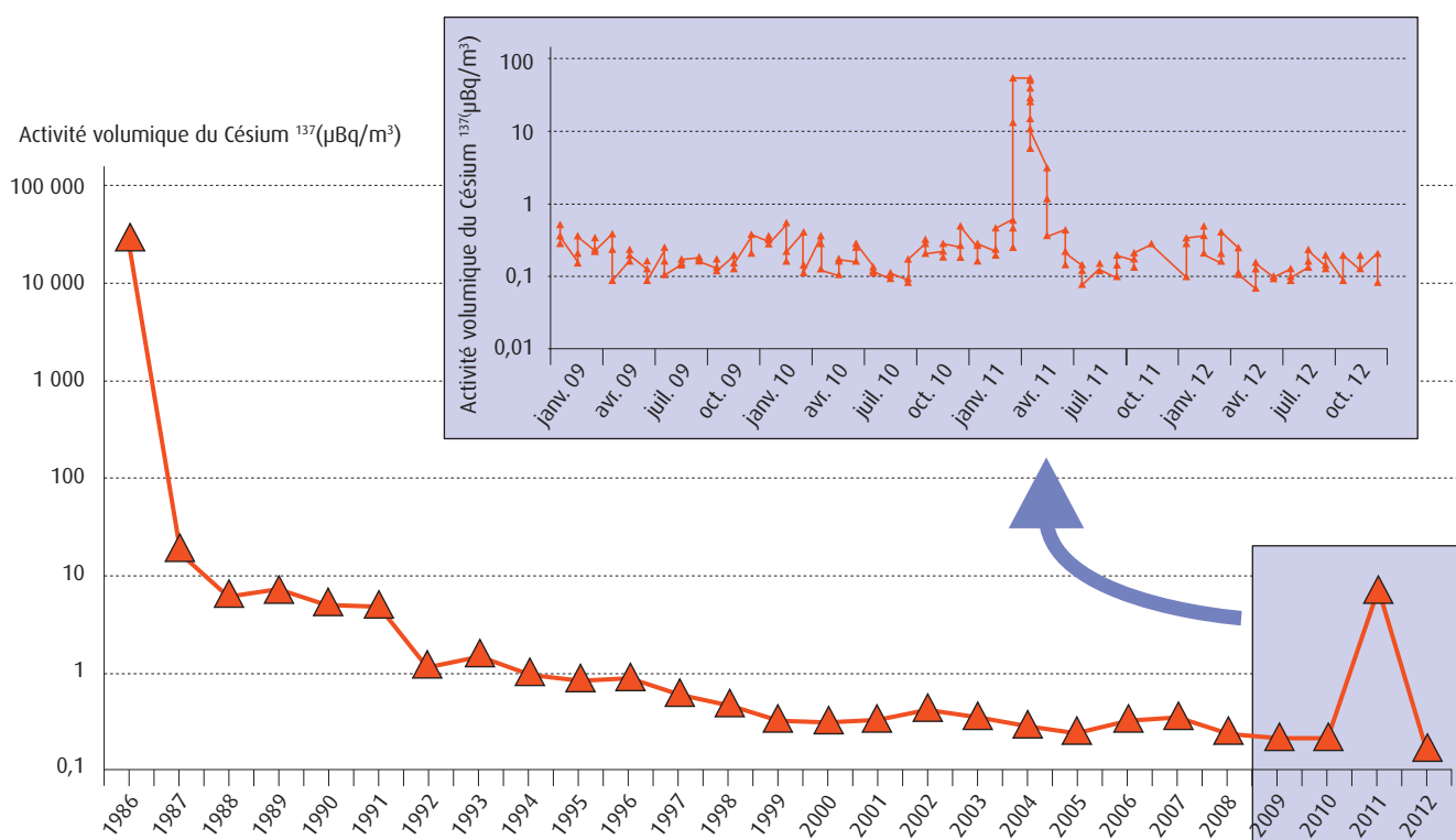
Figure 52 : évolution de l'activité volumique en ^{137}\text{Cs} dans l'air
