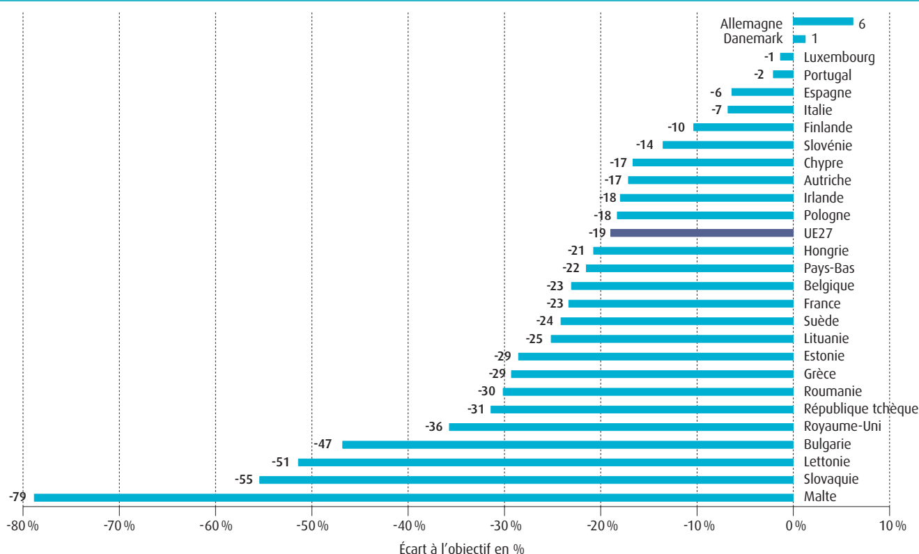
Figure 87 : écart vis-à-vis des objectifs de la directive NEC pour les émissions de COVM des 27 pays de l'Union européenne en 2010
