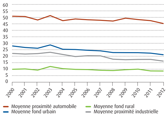
Figure 77 : évolution des concentrations en NO 2
