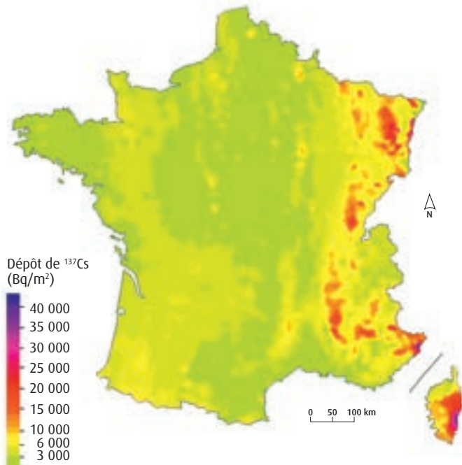
Figure 50 : activités surfaciques du ^{137}\text{Cs} potentiellement présentes dans les sols français en 2007
