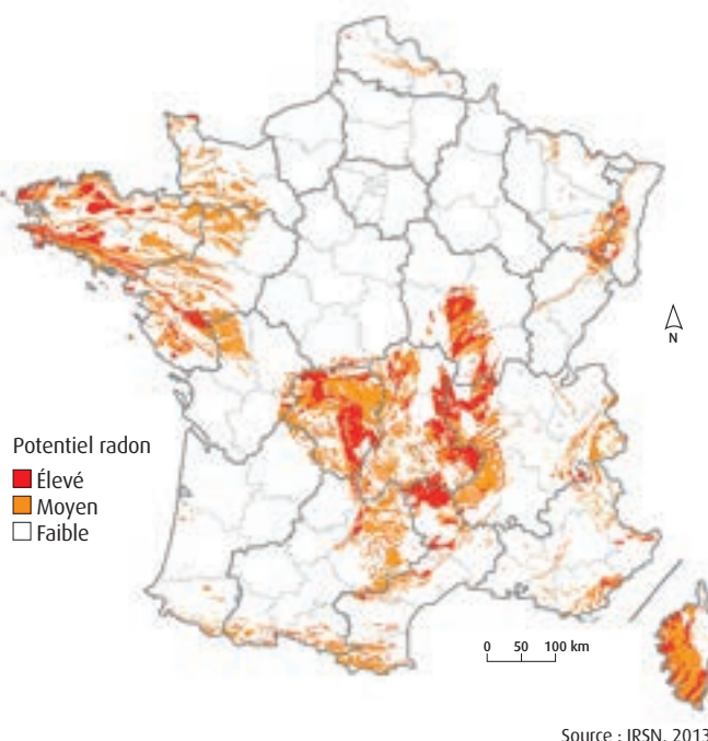
Figure 49 : potentiel radon des formations géologiques
