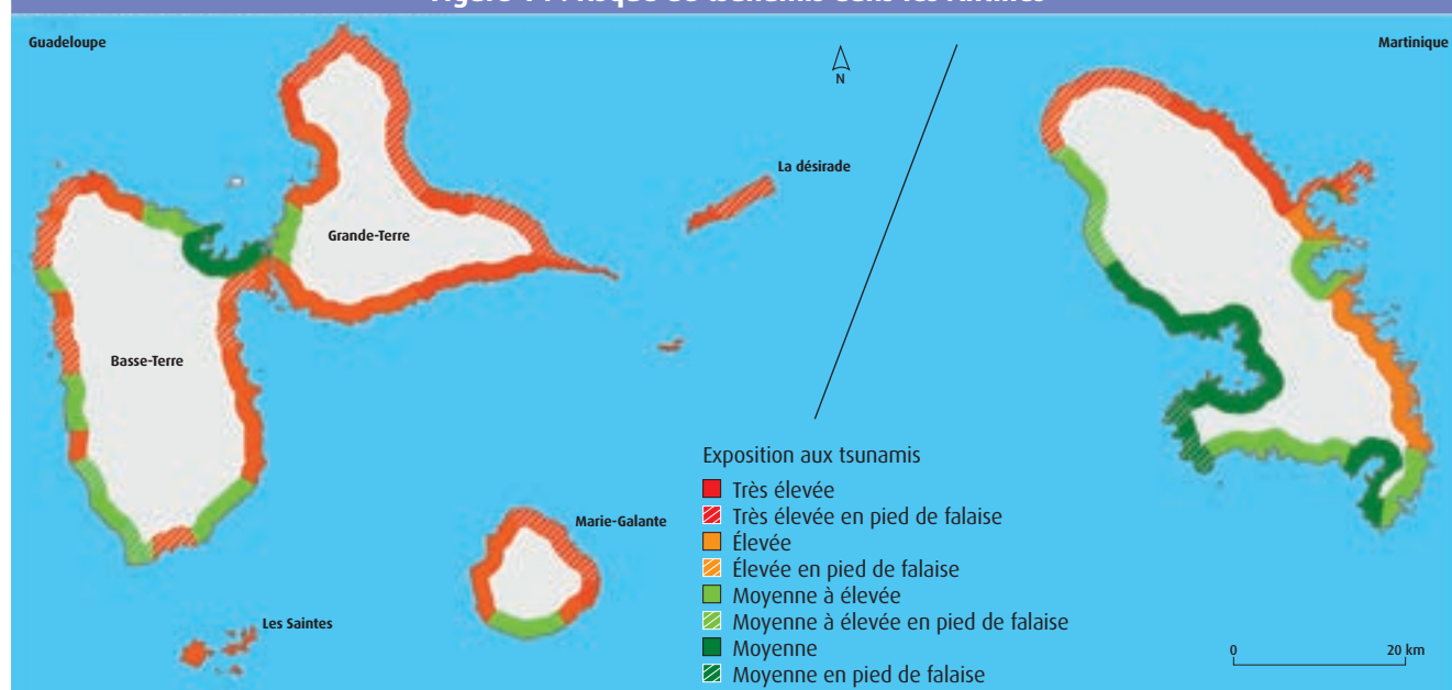
Figure 14 : risque de tsunamis dans les Antilles
