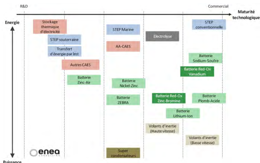
Figure 36. Niveau de maturité technologique des différentes méthodes de stockage électrique (Source : ADEME 159 )
