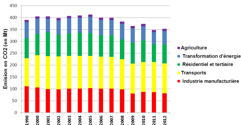
Figure 10. Evolution 1990 - 2012 des émissions de CO 2 par secteur (Cour des comptes d'après les données du CITEPA et ENERDATA)
