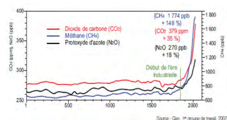
Figure 2. Concentrations atmosphériques de GES de l'an 1 à 2005.
