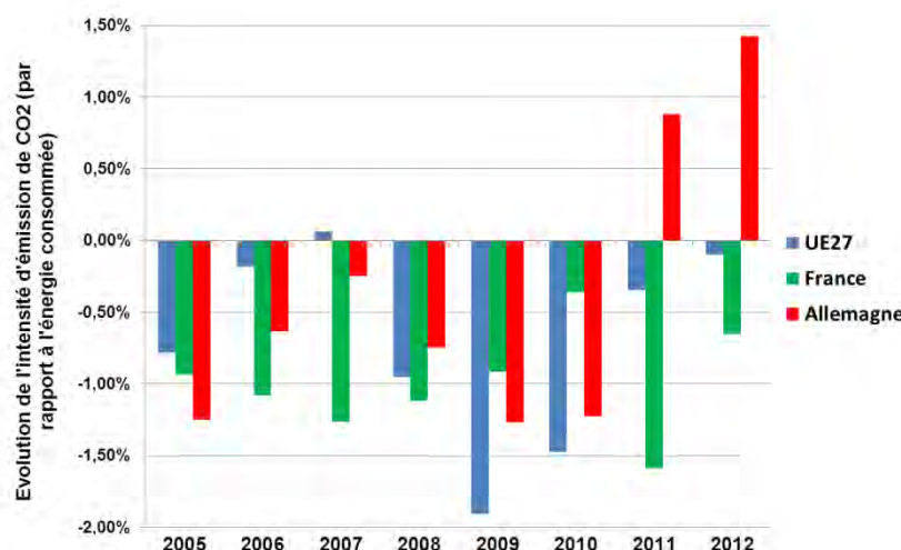
Figure 33. Evolution de l'intensité en émission de CO 2 de la consommation énergétique (variation du rapport des émissions sur l'énergie consommée). (Source : Enerdata 2013)
