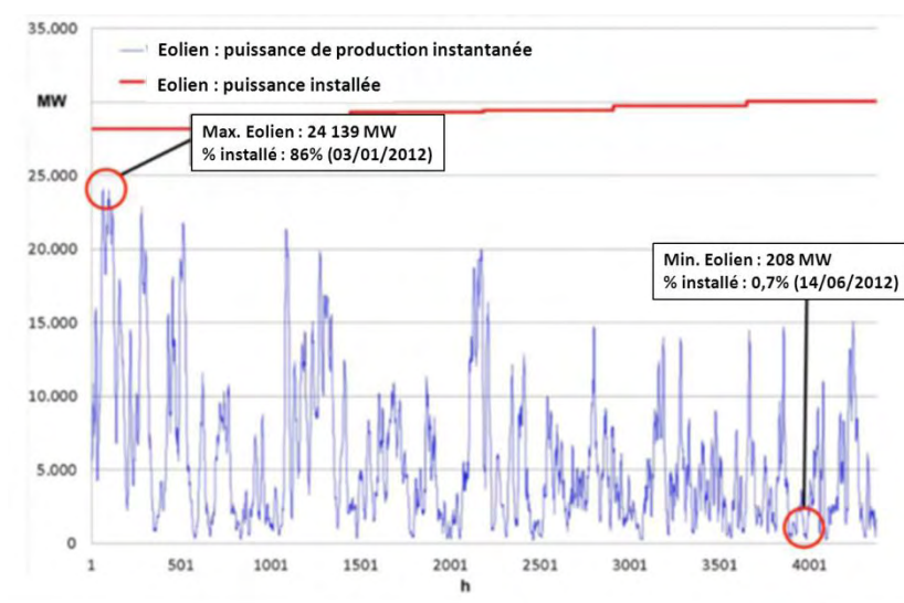
Figure 34. Production instantanée d'énergie renouvelable (éolien et photovoltaïque) en Allemagne, heure par heure pour les six premiers mois de 2012. En trait continu rouge, la capacité totale installée. (Source : Cour des comptes, d'après World Energy Council, Dr Leonhard Birnbaum, Monaco, 7 Novembre 2012)
