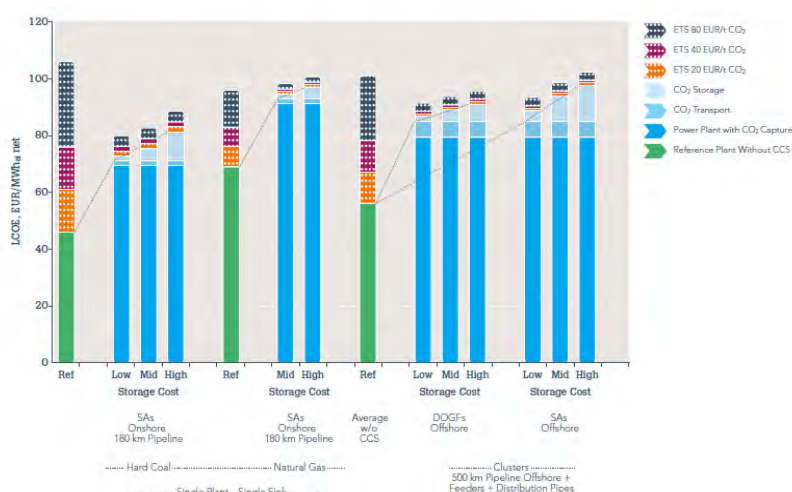
Figure 93. Le coût total de l'électricité (LCOE) pour des projets de CSC (barres bleues) comparées à des installations sans CSC (barres vertes) prenant en compte différents prix de stockage et avec une hypothèse d'un coût moyen du combustible. Source ZEP
