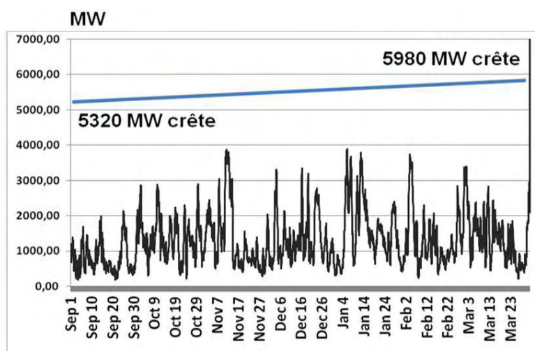
Figure 35. Production éolienne en France de septembre 2010 à mars 2011 (la courbe donne l'évolution heure par heure, ces valeurs étant extraites du site Eco2mix de RTE qui fournit ces données par ¼ heure) (Source : Hubert Flocard et Jean-Pierre Pervès 156 )
