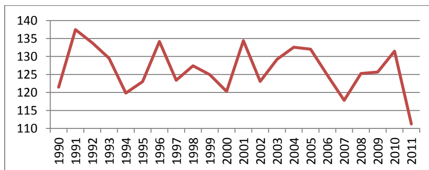
Figure 15. Logement-tertiaire : émissions de GES (en PRG) de 1990 à 2011 (données CITEPA, calculs Cour des comptes)
