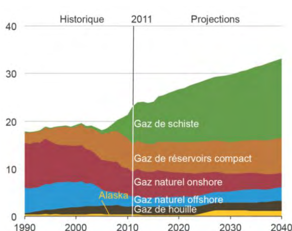
Figure 30. Production de gaz aux États-Unis 1990- 2011 et prévisions 2040 en « trillions de pieds cube » (Source : Annual Energy Outlook, avril 2013)
