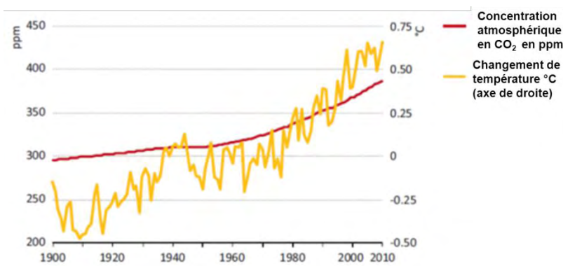
Figure 1. Evolution de la température moyenne mondiale (en jaune) au regard de l'évolution de la concentration atmosphérique de CO 2 . Source: Cour des comptes d'après "Redrawing the energy-climate map. World Energy Outlook Report, June 10th, 2013".
