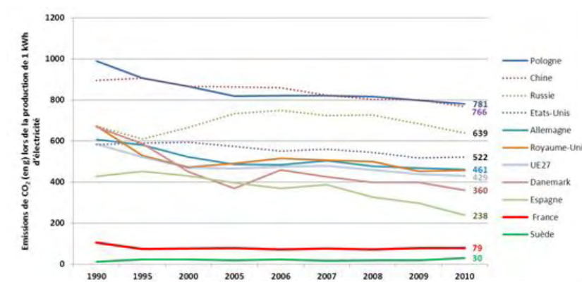
Figure 6. Emissions de CO 2 lors de la production de 1 kWh d'électricité (Source : Cour des comptes, d'après AIE/OECD, CO 2 emissions from fuel combustion Highlights, 2012 Edition)
