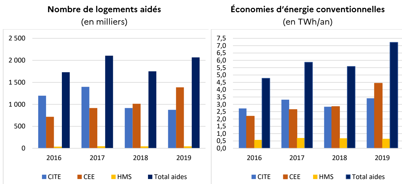
Graphique 1 : nombre de logements aidés et économies d'énergie associées
