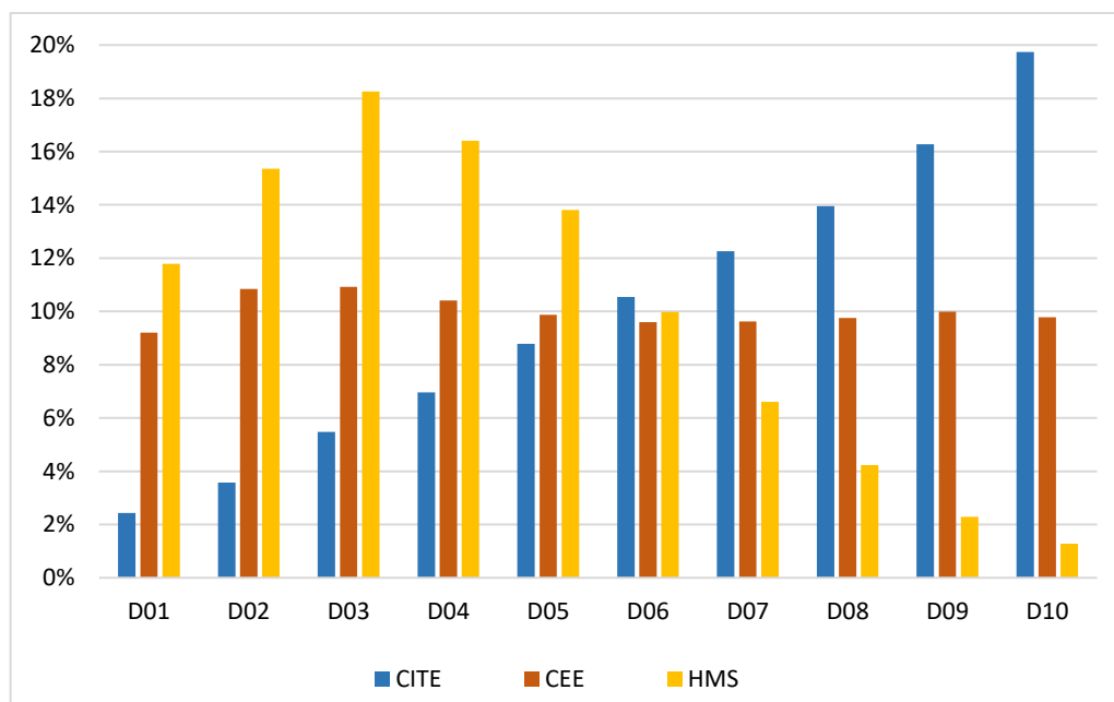
Graphique 14 : économies d'énergie, entre 2016 et 2019, par déciles de revenus selon le type d'aide
