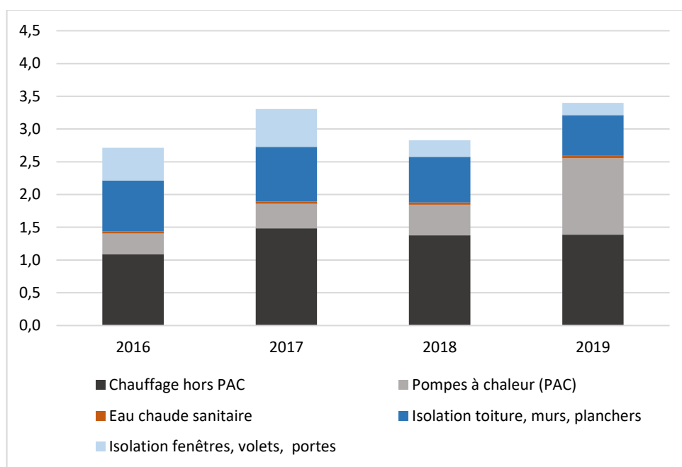
Graphique 4 : économies d'énergie par type de gestes aidés dans le cadre du CITE (en TWh/an)
