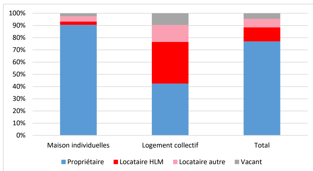
Graphique 11 : économies d'énergie 2016-2019, par statut d'occupation du logement
