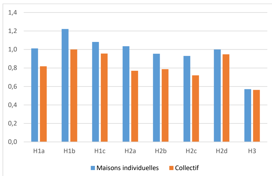
Graphique 9 : économies d'énergie rapportées à la surface habitable, entre 2016 et 2019, par type de logement et zone climatique En MWh/an pour 100 m 2
