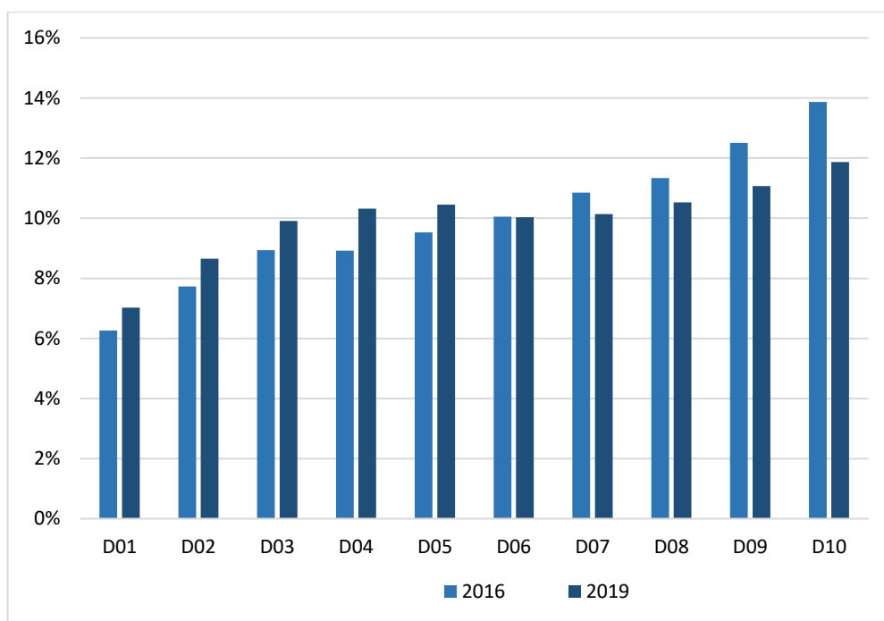
Graphique 12 : économies d'énergie 2016 et 2019 des CITE, CEE ou Habiter mieux, par déciles de revenus disponibles par unité de consommation
