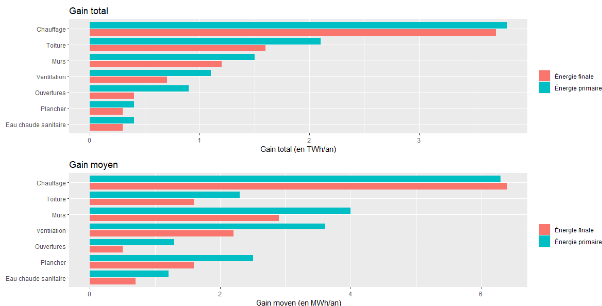
Graphique 13 : gains énergétiques par geste selon le poste rénové
