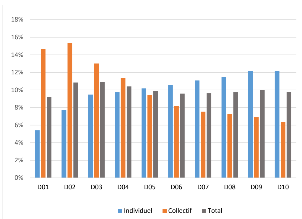
Graphique 15 : économies d'énergie des CEE, entre 2016 et 2019, par déciles de revenus et type de logement
