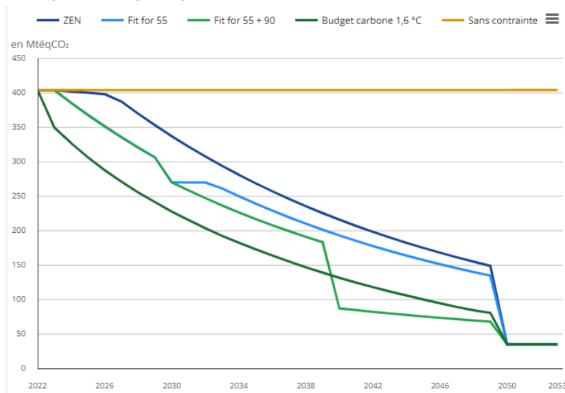
GRAPHIQUE 9 : FLUX BRUTS ANNUELS D'ÉMISSIONS DE GAZ À EFFET DE SERRE (GES), SELON LES DIFFÉRENTS SCÉNARIOS VERS LA NEUTRALITÉ CARBONE
