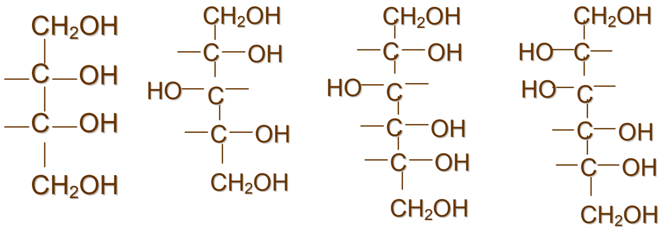
Erythritol
