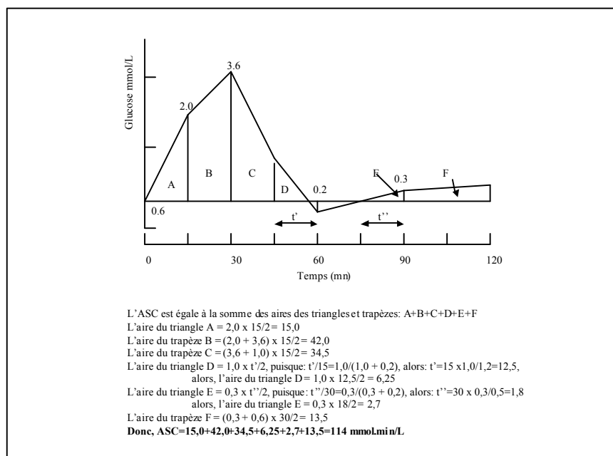
Figure 1 : Illustration du calcul d'une aire sous la courbe (ASC) de réponse glycémique (d'après FAO/WHO, 1998)
