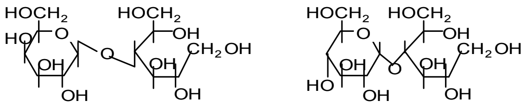
Lactitol
