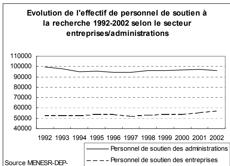
Graphique 5 : Évolution des effectifs de personnel de soutien par secteur
