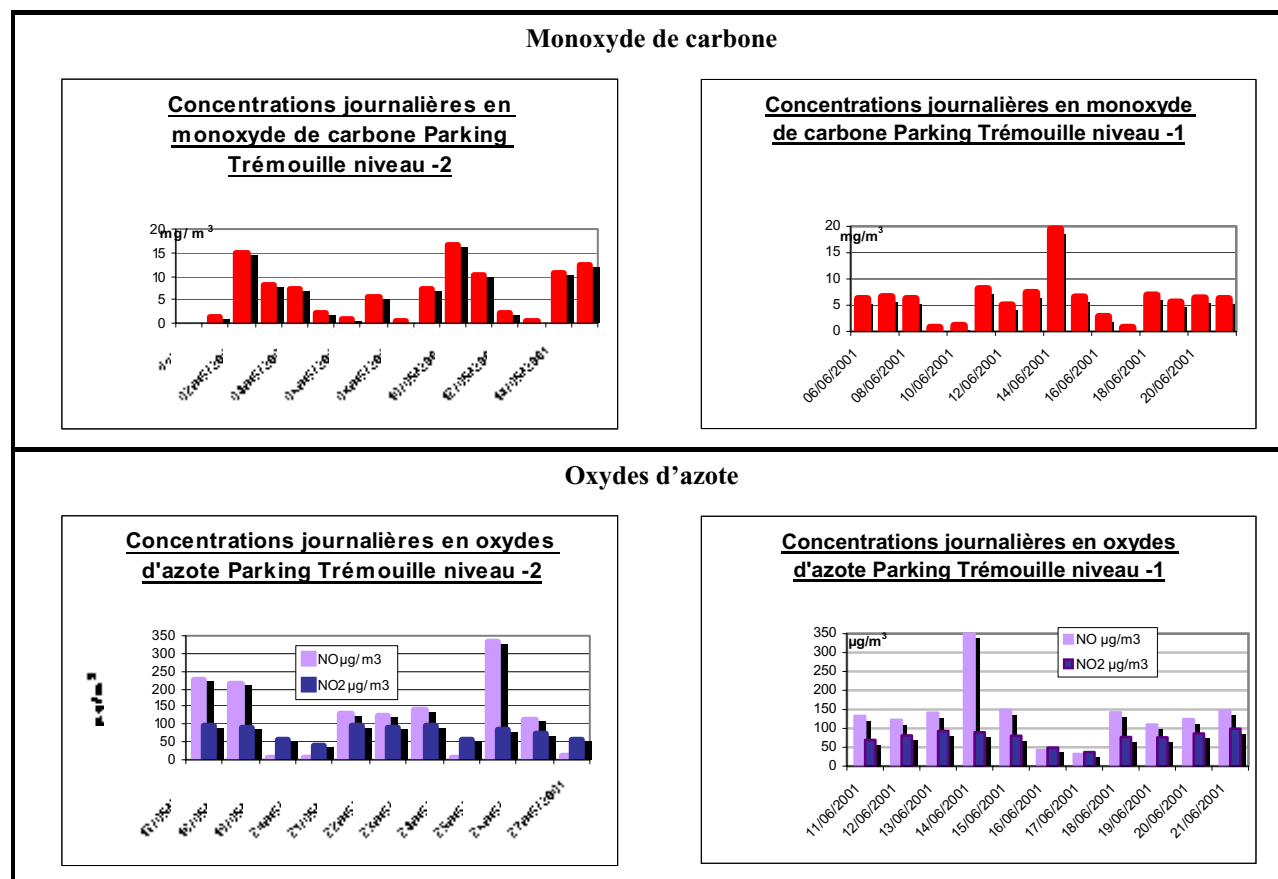
Figure 2 : Graphe des concentrations en CO et NOx dans un parking dijonnais (extrait de [Atmosf'Air Bourgogne, 2001])
