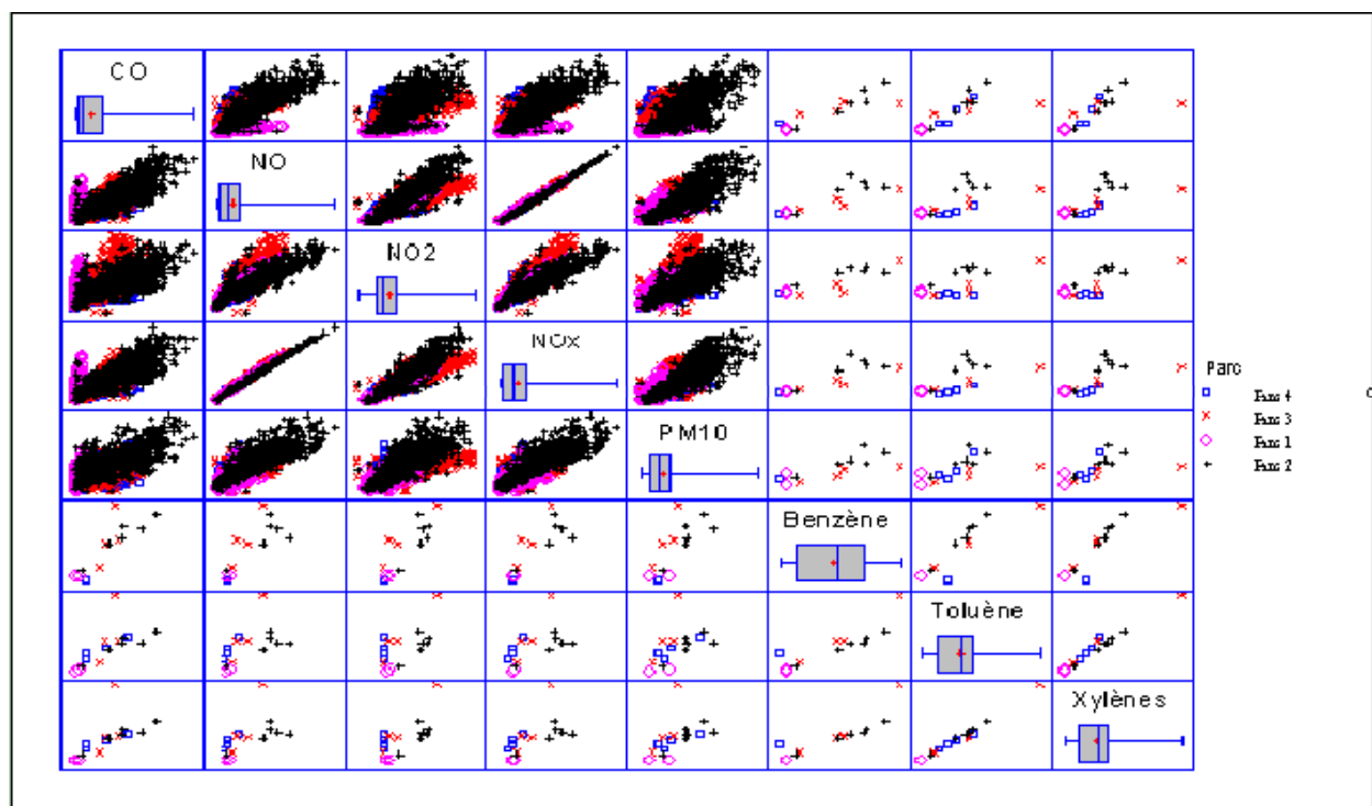
Figure 10 : Nuages de points des corrélations des données sur 30 minutes
