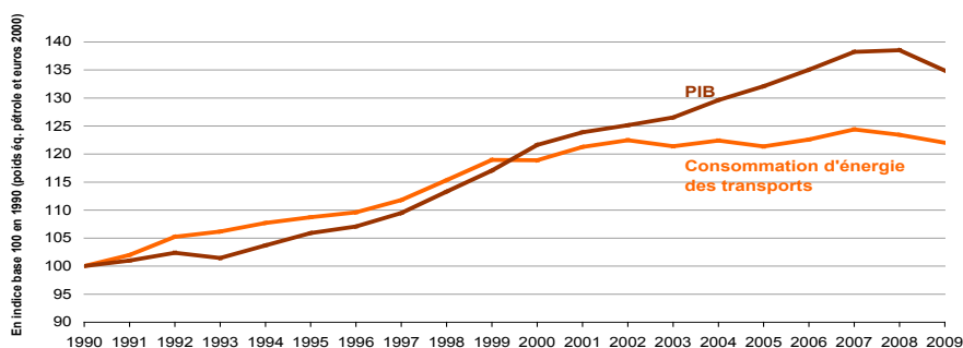
Graphique 71 : consommation d'énergie des transports et PIB en France (en indice base 100 en 1990, poids éq. pétrole et euros 2000)
