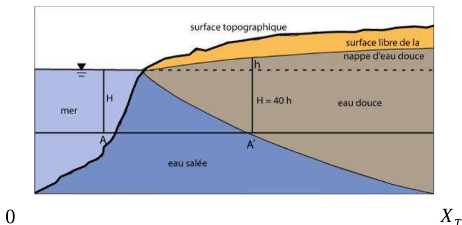
Figure IV.6: Coupe schématique perpendiculaire au littoral selon Ghyben-Herzberg (extrait de Frissant et al., 2005).
