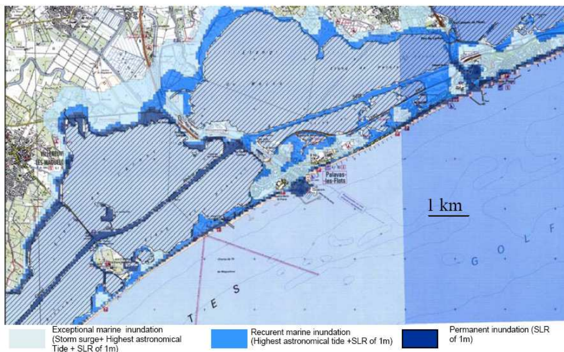
Figure IV.5: Scénario de tempête exceptionnel en 2100 basé sur l'hypothèse d'une tempête de type novembre 1982 et une hypothèse de 1m d'élévation du niveau marin. Source Vinchon et al. (2010).
