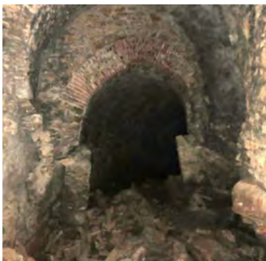
Bombement, affaissement des piédroits. Déstabilisation de la voûte en cours (Galerie « Forge » à Bessèges) source 4 photos : Antea Group – CC Cèze Cévennes
