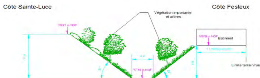
Schéma type du cavalier minier en contrebas de la rue des Festeux
