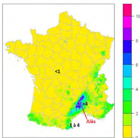
Débit ( \text{m}^3/\text{s} ) quinquennal pour une surface de 1\text{ km}^2 Source : modèle SHYPRE développé par IRSTEA
