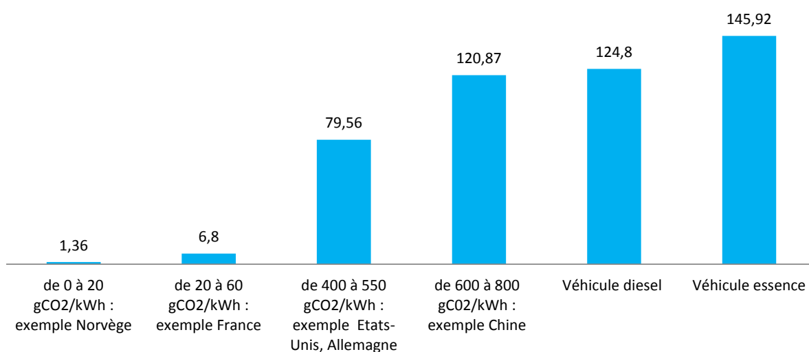
Graphique 25 – Ordre de grandeur des émissions de CO 2 en grammes pour un km parcouru en fonction des émissions de différents mix de production d'électricité 1
