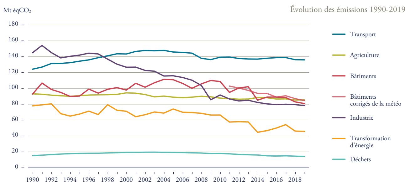
Figure 2a – Tendance dans les émissions sectorielles en France
