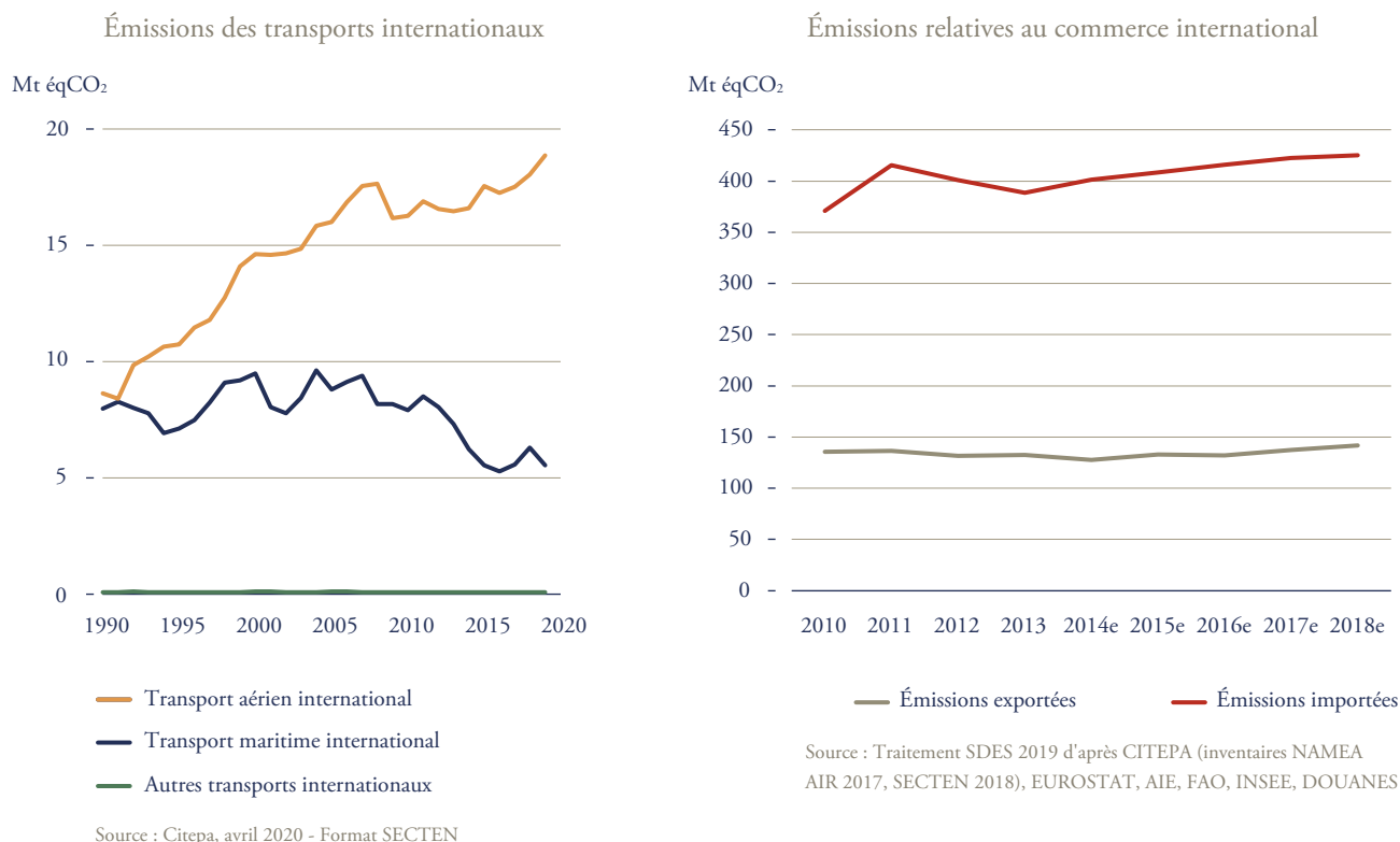
Figure 3 – Tendances des émissions relatives aux échanges internationaux
