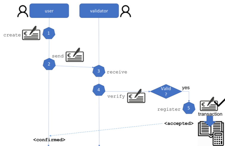
Figure 14 - Cycle de vie d'une transaction avec un validateur
