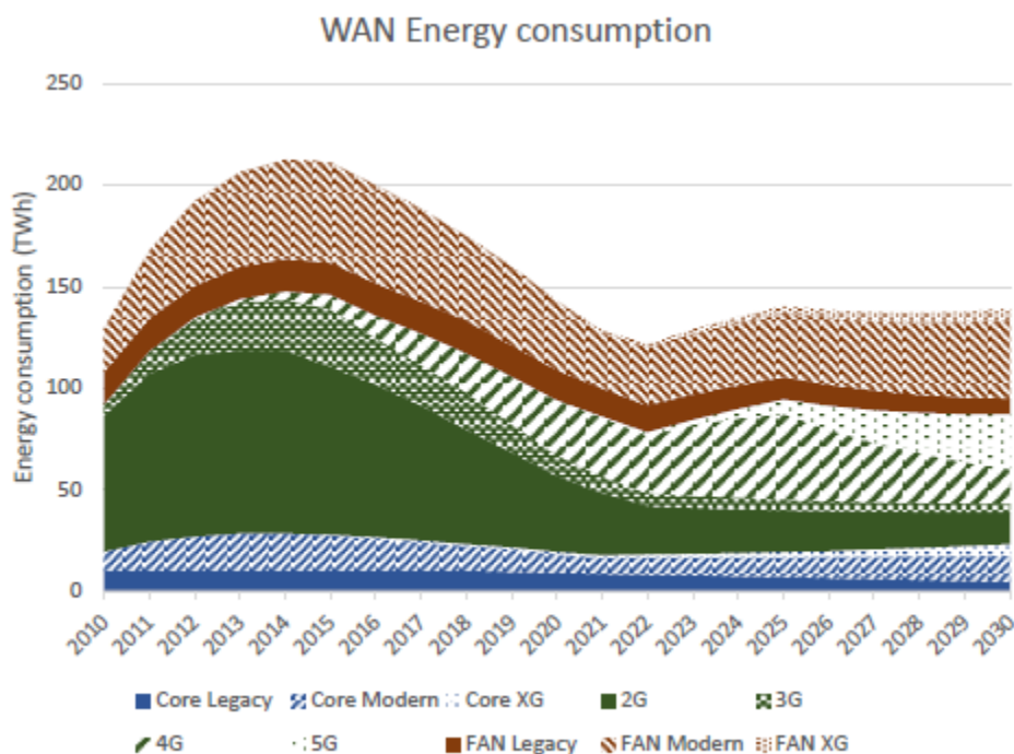
Figure 45 - Consommation énergétique des réseaux WAN au niveau mondial selon les projections de l'EDNA 154
