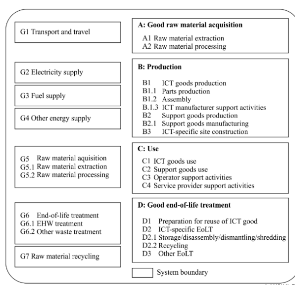
Figure 4 - Les limites du système de produits pour l'ACV des biens, réseaux et services liés aux TIC 56
