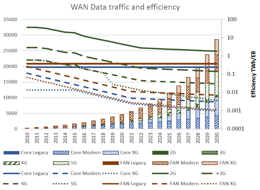
Figure 41 - Trafic de données WAN et efficacité énergétique au niveau mondial par catégorie de composant selon le modèle de l'EDNA 176 . Les unités en ordonnées gauche sont des Exabits (EB)
