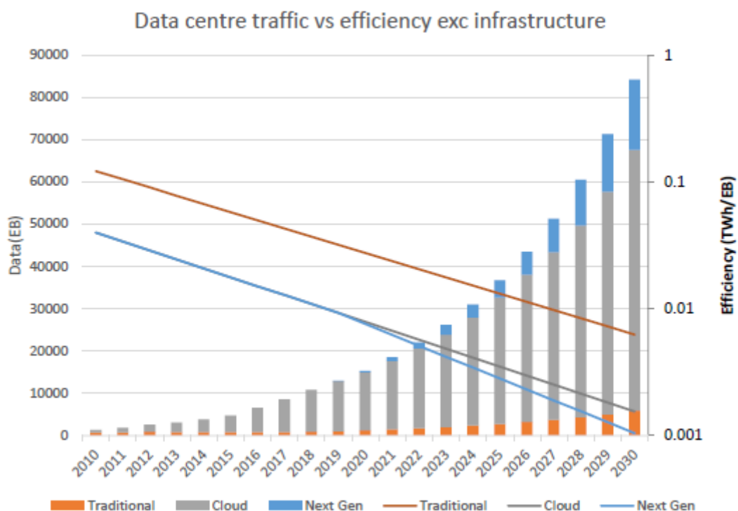
Figure 46 - Trafic de données dans les datacenters au niveau mondial et efficacité énergétique 176
