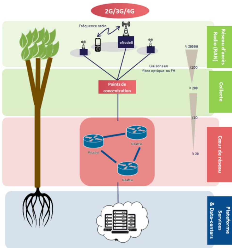
Figure 13 - Illustration de l'architecture d'un réseau mobile 2G/3G/4G et analogie avec un arbre – Plateforme de travail « Pour un numérique soutenable » Atelier « Façonner les réseaux pour un numérique soutenable » - Novembre 2020
