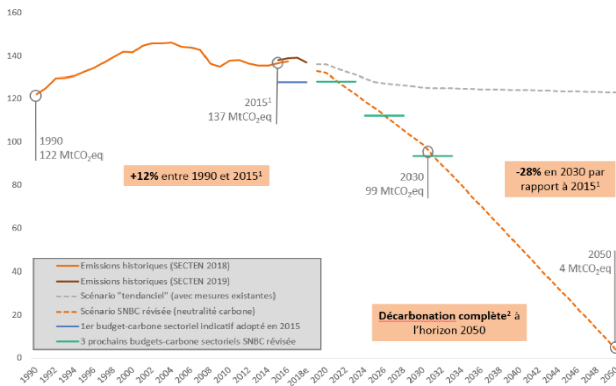
Graphique 5 – Historique et projection des émissions du secteur des transports entre 1990 et 2050 (en MtCO 2 eq)
