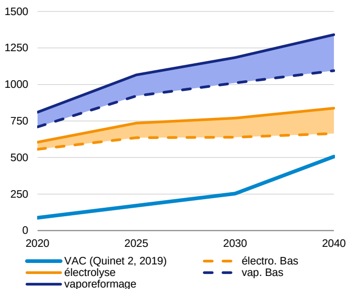
Graphique 19 – Coût d'abattement ajusté à la VAC des véhicules hydrogène
